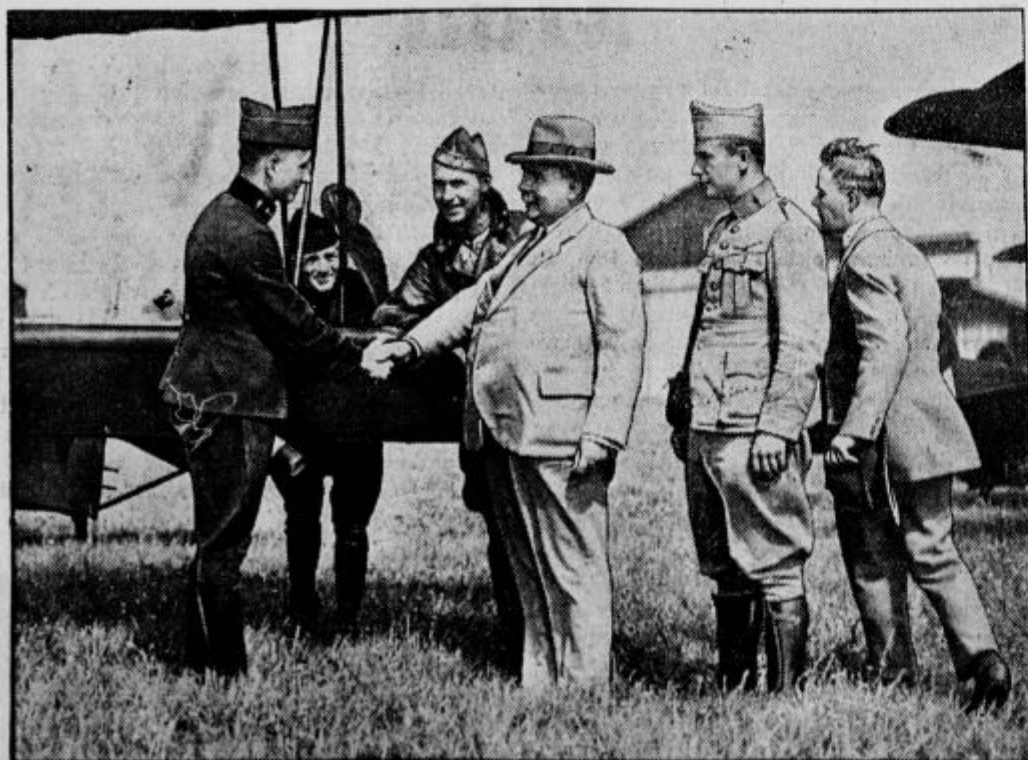
Holandski izdelovatelj dežja pred svojim letalom. Na Holandskem so nedavno vzbudili veliko pozornost poizkusni inženjerja Veraarta, ki se je dvignil z letalom, na katerem je bil naložen zdrobljen led, ki ga je nato stresal in tako napravil umeten dež. Veraarta so sedaj povabili v Berlin, da tam ponovi svoje poizkuse, ker njegovi metodi prisojajo veliko važnost.
