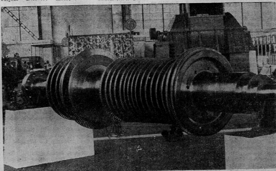
V »Jugoturbini« izdelani rotor, namenjen za parno turbino zagrebške toplarne, zbujajo na zagrebškem velesejmu veliko pozornost med obiskovalci (Foto: Igor Prešern)
