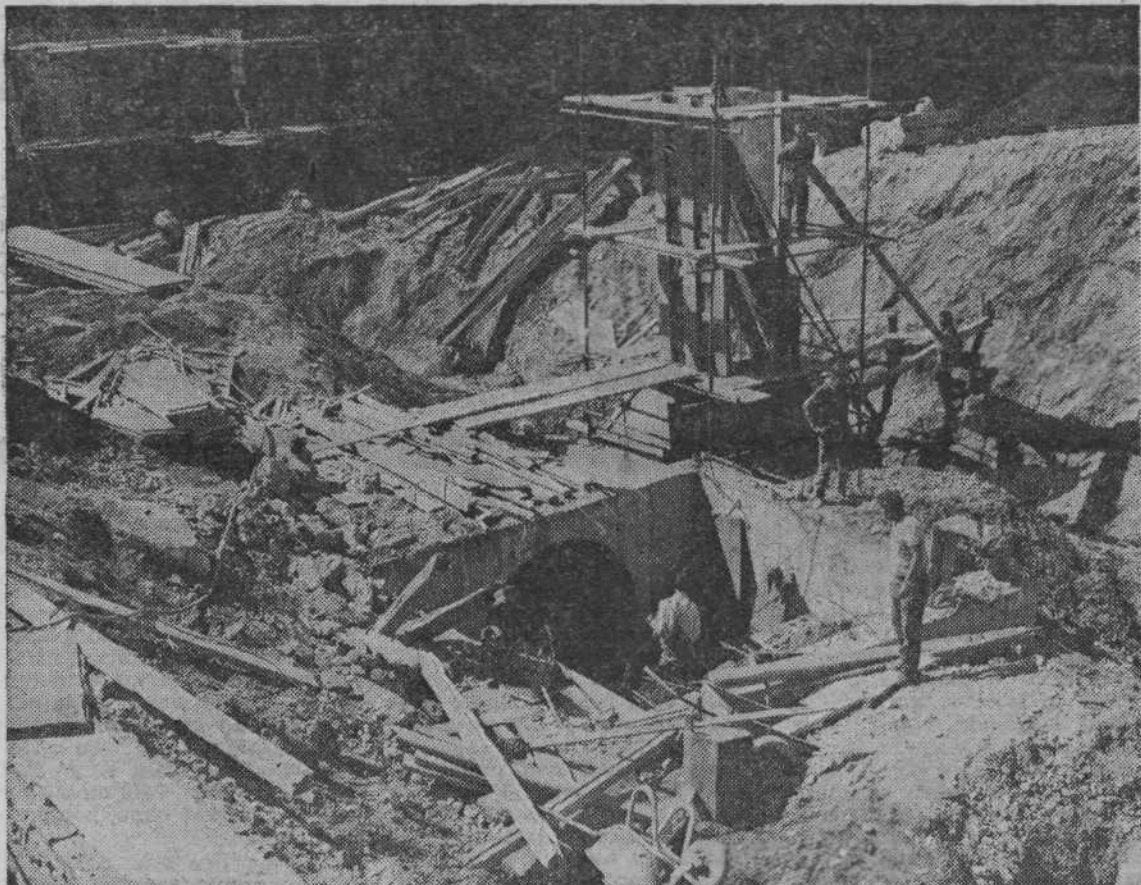
Spredaj eden od kolektorjev, za njim pa gradnja enega od nosilnih stebrov podhoda, ki so ga, zaradi zamud, pričeli postavljati pred rokom. V ozadju gradnja stene bodočega podhoda.
