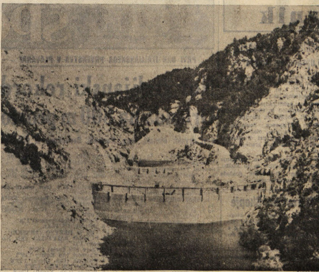
Veliki jez. Kruščica, ki bo zapiral umetno jezero s 120 milijoni kubnih metrov vode, sodi med največje objekte, ki jih je treba izgraditi na 50 km dolgem gradbišču hidrocentrale Senj. Gradbišče se razteza od Perušića v Liki do Grabova na obali Jadrana. Na sliki: temelji Kruščice.
