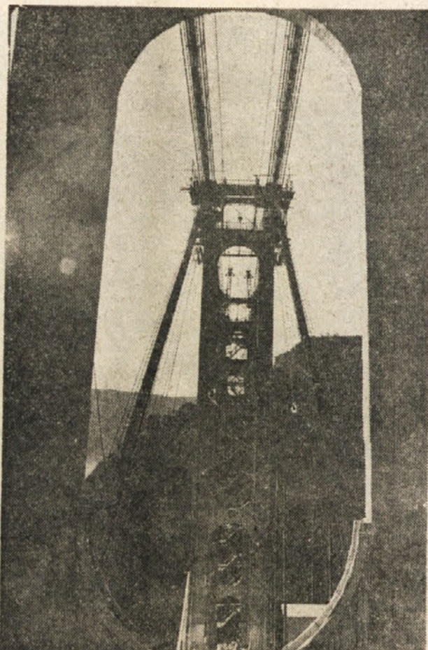
POGLED SKOZI OGRODJE — V votlem delu lokov bo pod cestiščem speljan jugoslovanski naftovod, razen njega pa vodovod ter električni in poštni vodi.
