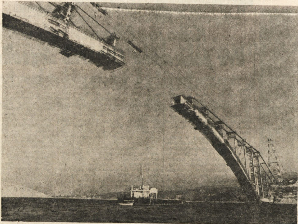
KRAKA BETONKEGA LOKA SI RASTETA NASPROTI — Prej kot v dveh tednih bo spojen še drugi, daljši lok na mostu, po katerem bo s kontinentalno peljala cesta čez otoček Sv. Marko na naš največji jadranski otok. Na sliki v sredini plavajoča gradbena ploščad.
