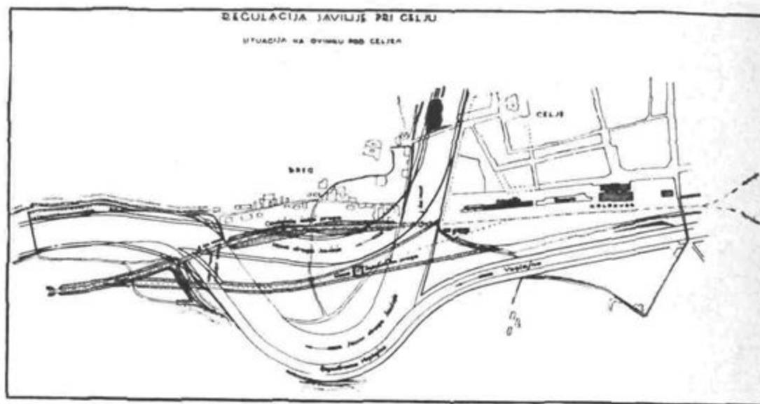
Regulacijski načrt Savinje pri Celju
