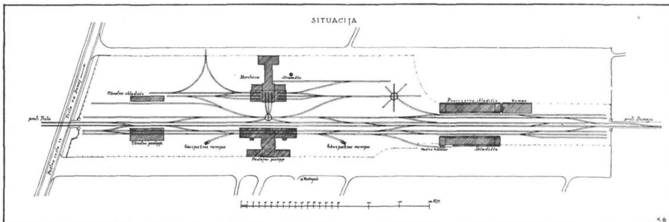
Tloris kolodvora l. 1849.
