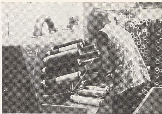
Stroj za odvijanje predpreje iz flyerskih cev v predilnici bombaža. Naredili so ga v naši mehanični delavnici.
