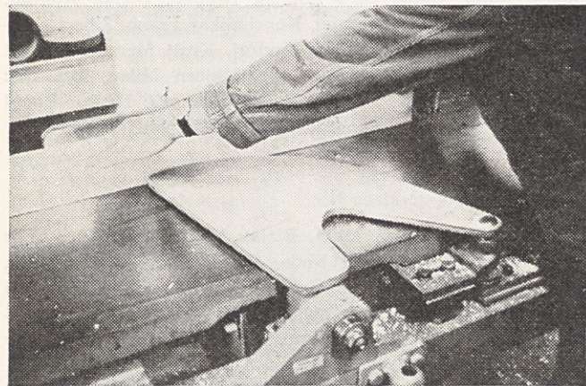
Zaščitna plošča nad noži poravnalnika varuje roke mizarja
