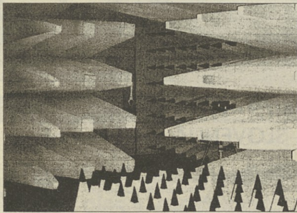
V takšnih studijih preizkušajo zvočnike: to so zvočno povsem izolirane komore
