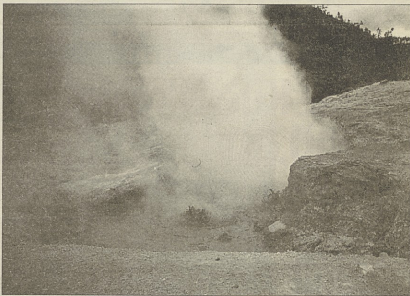
Sikajoča para na planoti Dieng (Foto: Marija Demšar)
