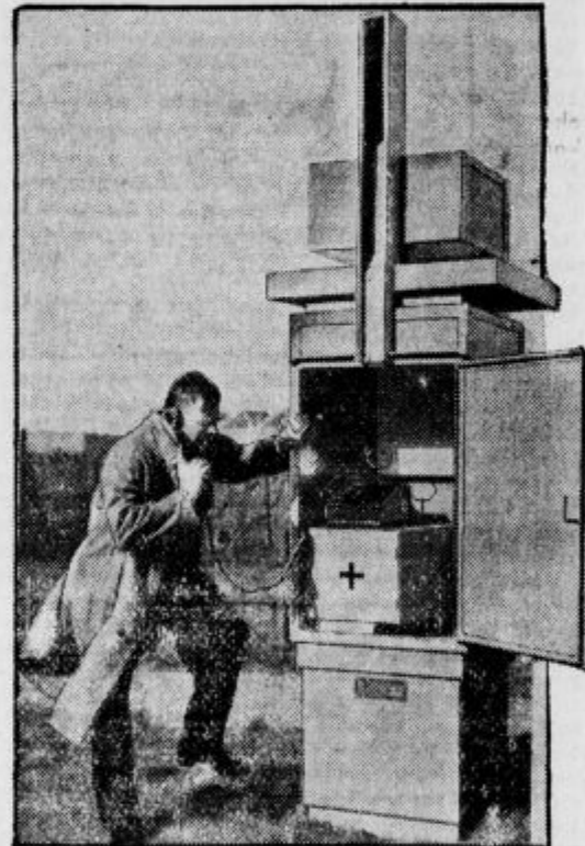
Na Holandskem bodo postavili takšne-le rešilne stanice na vseh važnejših cestah. Ponesrečenec bo v njih našel vse potrebno za prvo pomoč, obenem bo lahko tudi telefoniral po zdravnika, po policijo ali po ognjegase
