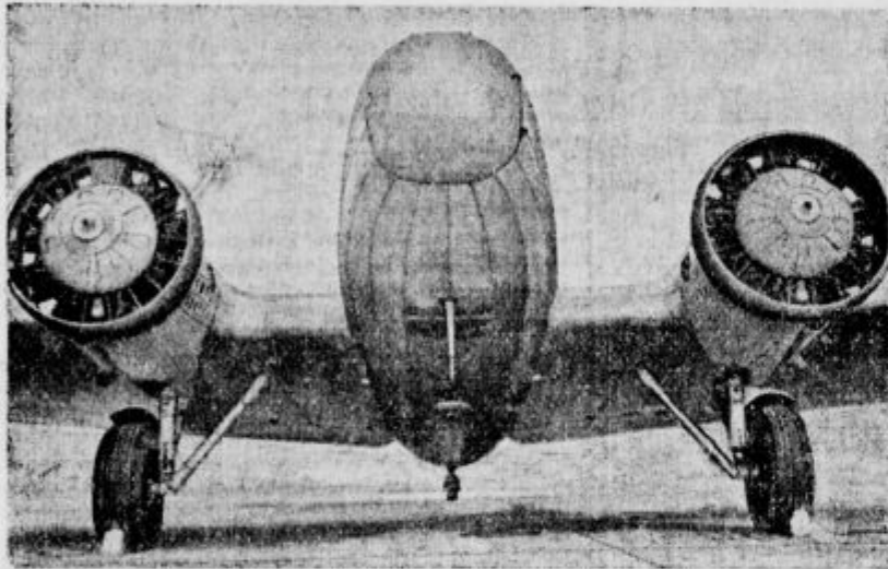
Ameriško letalo tipa Boeing 247, ki ga uporabljajo na prekoceanski progi in leti s hitrostjo 275 km. Tudi evropske promet. družbe so si nabavile več takšnih letal
