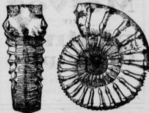
Slika. 1. Lična hišica amonita: prva slika na levi kaže pogled od spredaj, druga na desni pa od strani.
