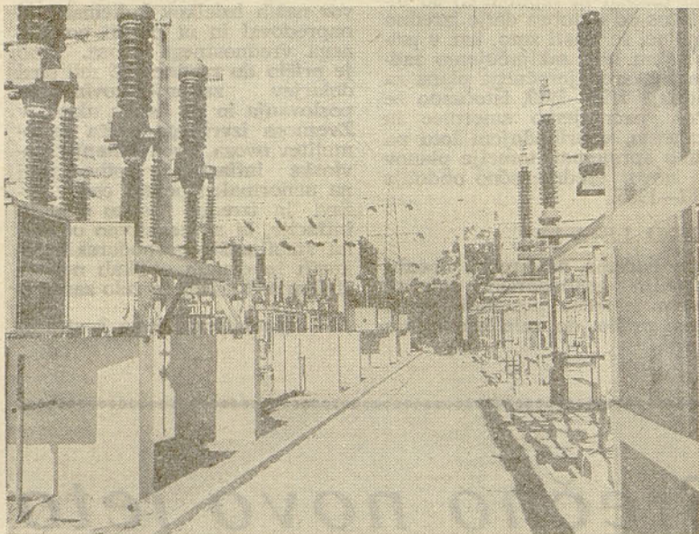
Nova trafopostaja Štore II
