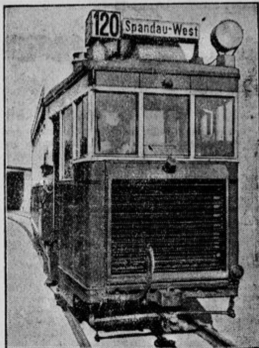
Cestno-železniški voz z bencinskim motorjem; take vozove uporabljajo v Berlinu na manj prometnih progah, kjer ni električne napeljave.
