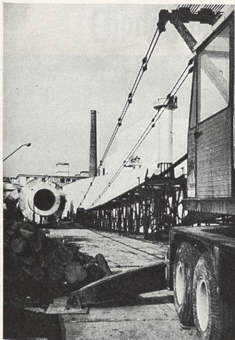
Italijansko dvigalo firme »F. Midolini« je sestavljeno in čaka na začetek dviganja prvega segmenta
