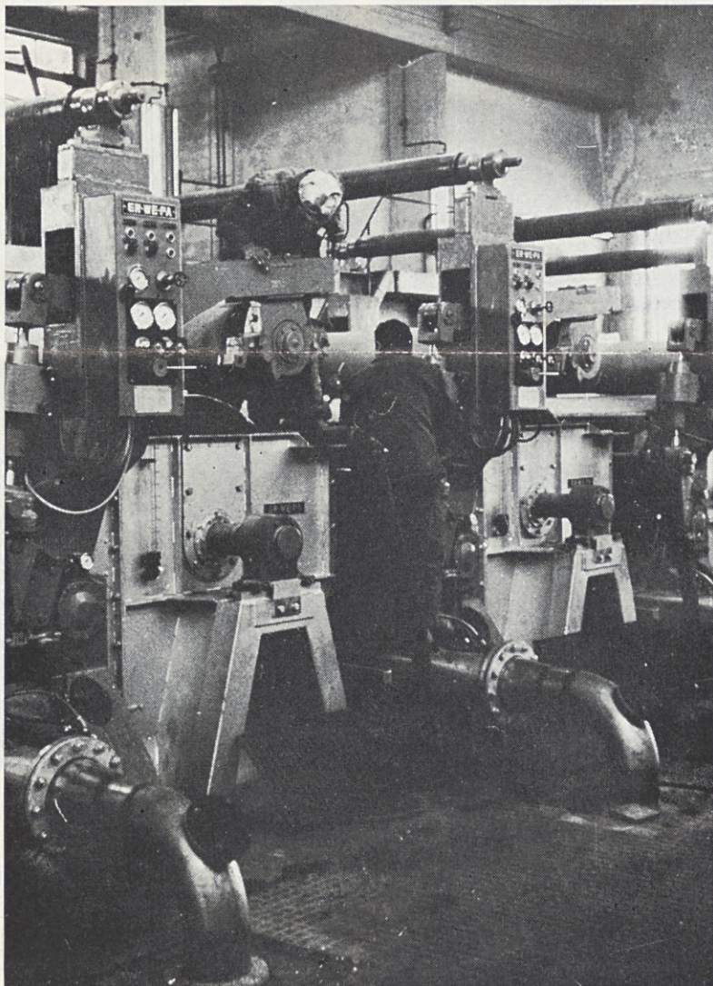
Čiščenje natočnih banj ob prehodu na izdelavo novega izdelka
