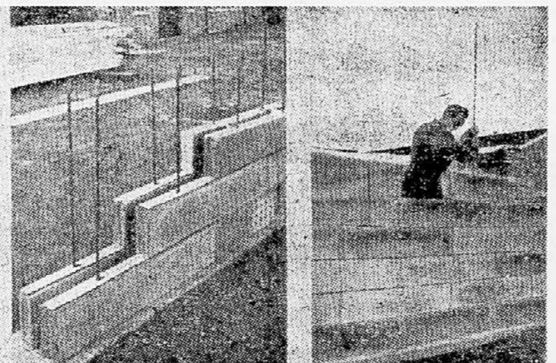
Neka angleška gradbena tvrdka je patentirala nov izum. Gre za posebno vrsto opeke, ki se nataka na jeklene palice, tako da ni treba zidati več z malto. Taka gradnja je veliko hitrejša, razen tega pa je mogoče zgradbo s takim zidom porušiti in prestaviti brez težav. Enodružinska hiša se more postaviti s to opeko v 24 urah.
