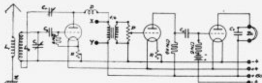
Shema trielektronskega radioaparata, prirejenega tudi za električno podajanje gramofonske glasbe. L_1 = 15 ovojev, L_2 = 65 ovojev, c_1 = 500 cm, c_2 = 500 cm, c_3 = 300 cm, c_4 = 5000 cm, c_5 = 2000-10.000 cm, R = 30 Ohm, P = 5 M \Omega
