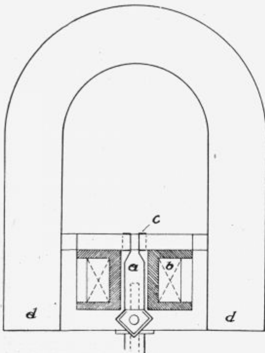
Shematična slika elektromagnetne gramofonske doze.
