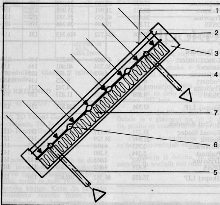
Shema ploščatega kolektorja:
