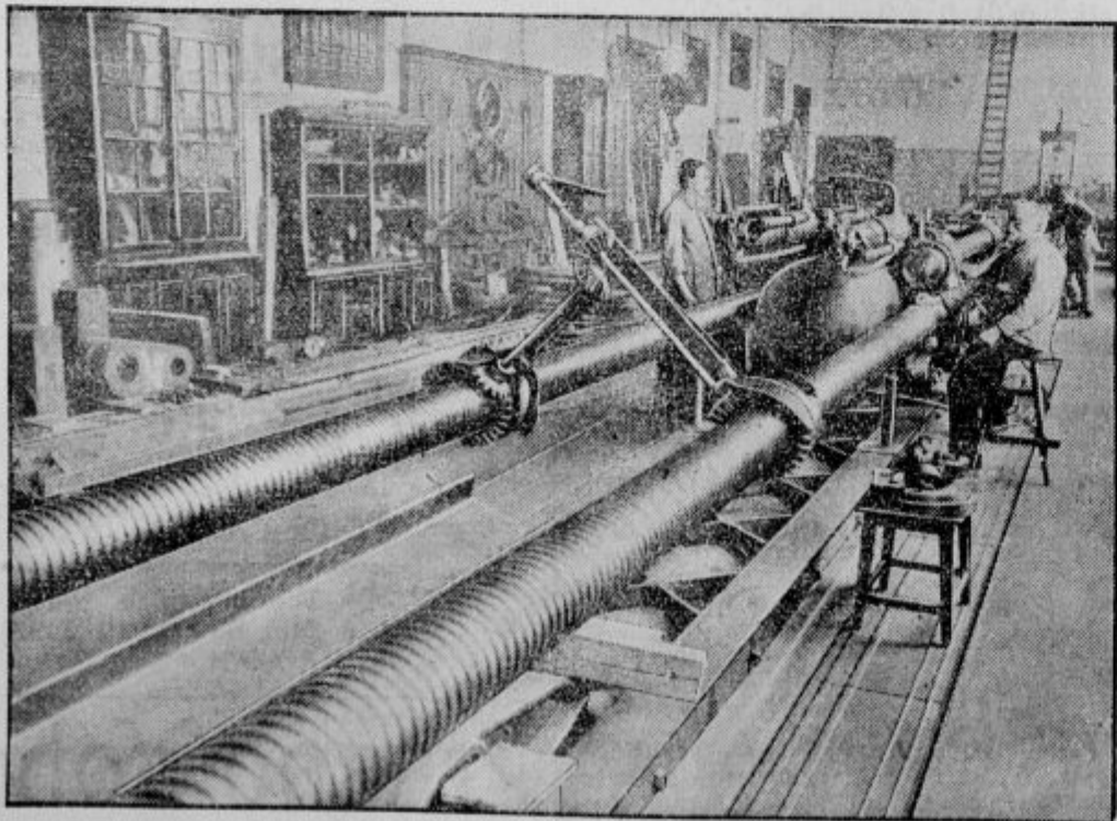
Stroj za lomljenje in trganje, s katerim izvršuje svoje preizkuse nemški državni urad za preizkušanje materiala. Na tem uradu, ki je istočasno največji znanstveni institut v Nemčiji, vse izdelke človeških rok raztrgajo, zlomijo, razrežejo, zdrobe in sežgo, da tako doženejo trdnost in odpornost vseh mogočih snovi.
