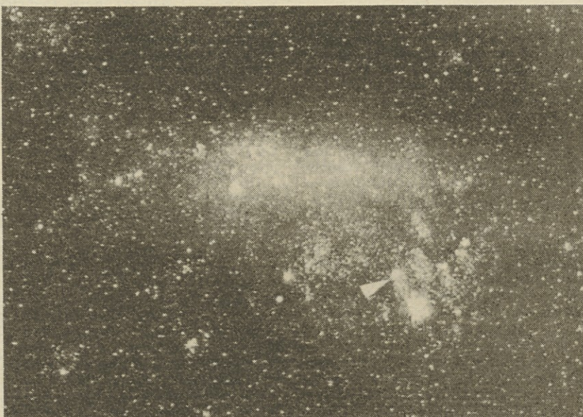
Puščica kaže supernovo v Magelanovem oblaku
