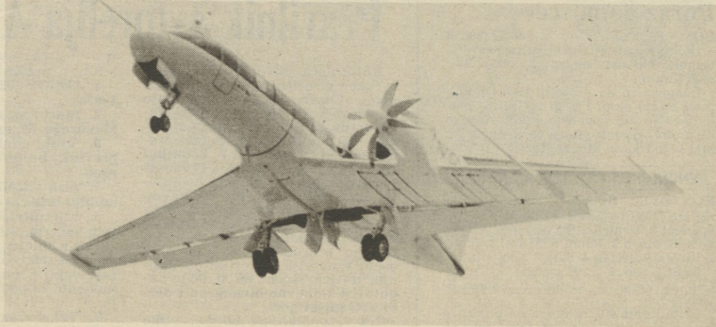
Enomotorni letal je na svetu mnogo, vendar je prototip na sliki svojevrsten. Gre za reaktivno letalo, ki ima na krilu motor z novim tipom propelerja, ki naj bi omogočil najmanj 20-odstotni prihranek goriva. (Telefoto AP)
