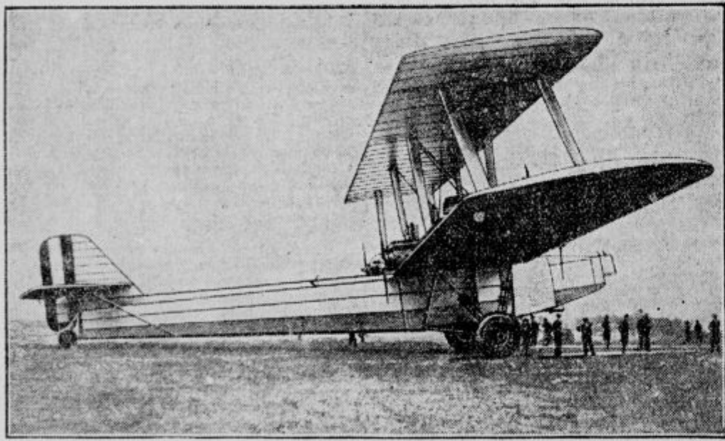
Največje letalo na svetu je »Caproni 6000«, ki ga sedaj v Milanu preizkušajo. Široko je 67 m, dolgo 28 m, visoko 11 m. Ima šest motorjev s 6000 konj. silami in doseže hitrost 210 km na uro.
