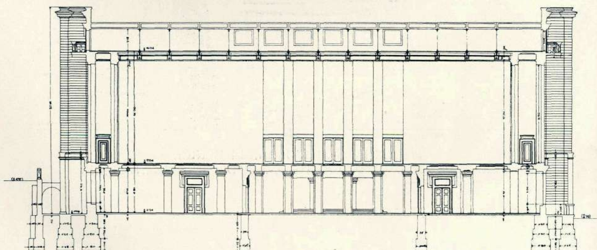
PREREZ A-B
