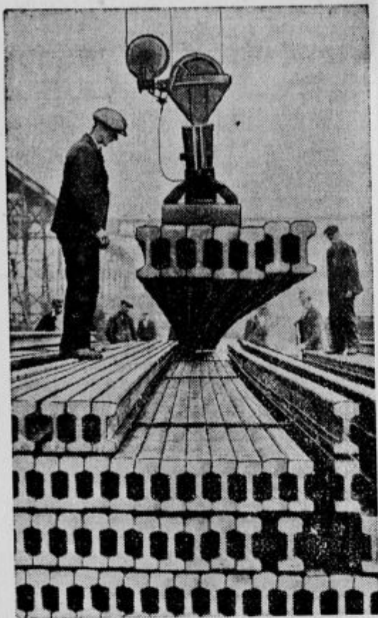
Elektromagnet dviga železniške tračnice, in sicer po sedem naenkrat! Elektromagnet, ki je pritrjen na žrvjavu, uporabljajo v working-tonskih jekelnah na Angleškem.
