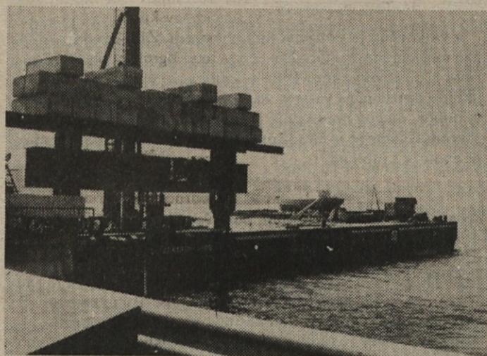
Meritve na poizkusnih pilotih za gradnjo podaljška kontejnerskega terminala.
