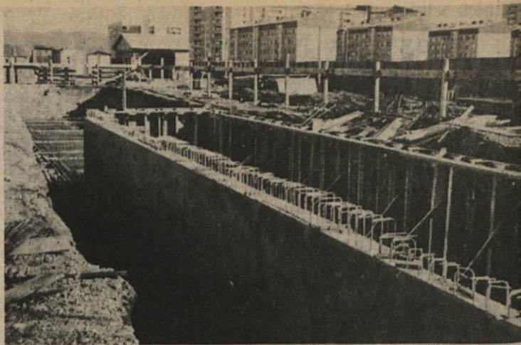
Prvi betoni so vgrajeni, čez nekaj mesecev bo stavba že pod streho.
