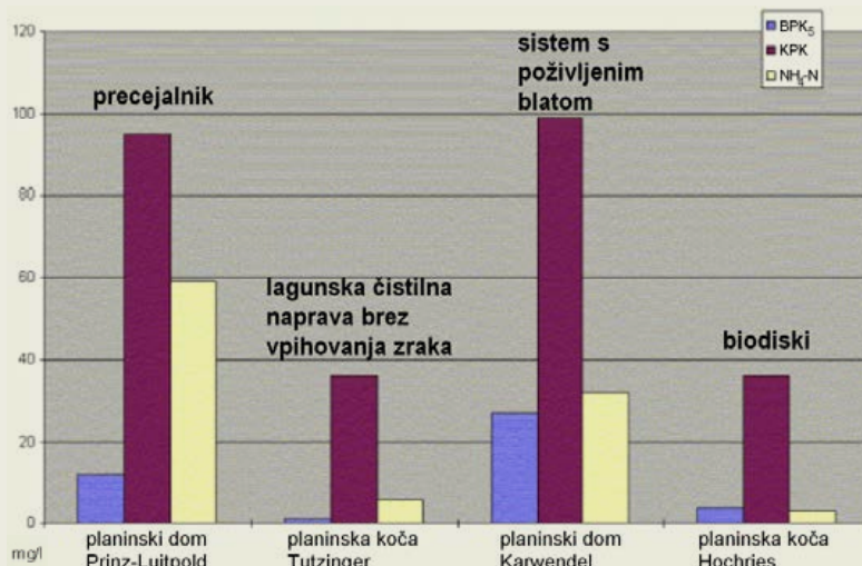
Diagram primerjave odtočnih vrednosti različnih čistilnih sistemov (1997/1999)
