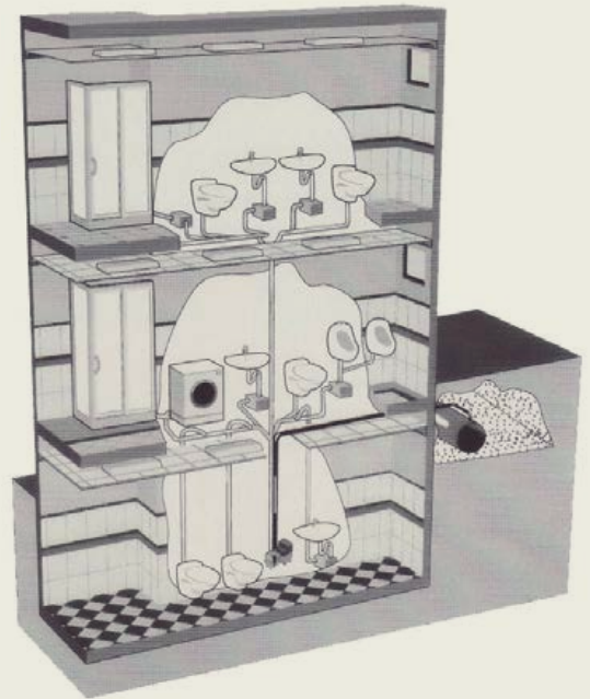
Shematski prikaz vakuumске naprave v zgradbi
