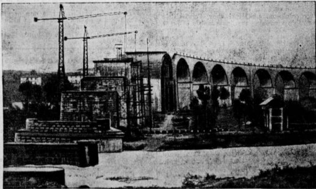
Ogromni železniški most pri Cuneo v Piemontu, ki bi bil po dograditvi najdaljši most na svetu, se je med gradbo 11. loka nenadoma zgrudil in pokopal pod seboj delavce. Devet delavcev je bilo takoj mrtvih, številne delavce so pa hudo ranjene odpeljali v bolnišnico.
