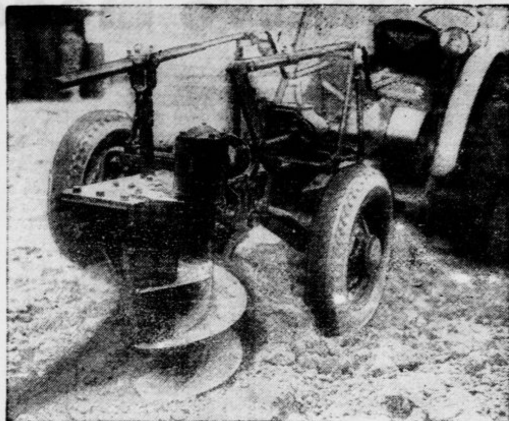
Najnovejši plug, izum nekega francoskega inženirja, ki orje zemljo s pomočjo posebne vijčne priprave in obenem seje
