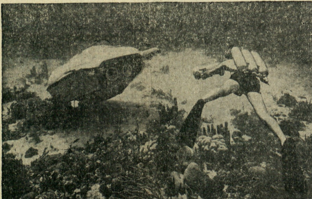
POTAPLJAJOČI SE KROŽNIK — Kap. Jacques-Yves Cousteau je izdelal napravo za raziskavanje vodnih globin, ki jo je imenoval "potapljajoči se krožnik". Sposobna se je gibati v globinah do 1000 čevljev. Doslej so jo uporabili za preiskave morskih globin v Sredozemlju in v Karibskem morju, nameravajo pa jo uporabiti tudi za raziskave pod arktičnim ledenim pokrovom.
