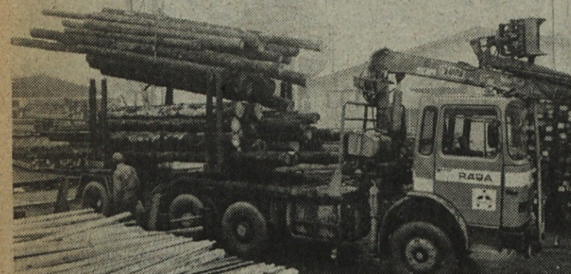
Dviganje hlodovine s tovornjaka z mostnim žerjavom
