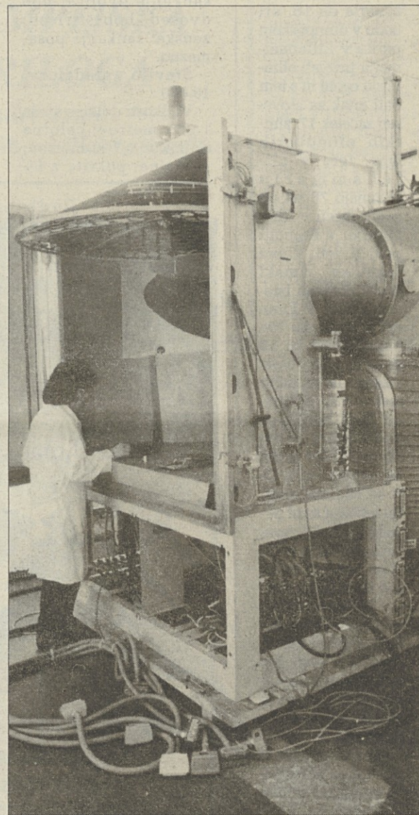
Stroj za vakuumsko metalizacijo avtomobilskih žarometov
