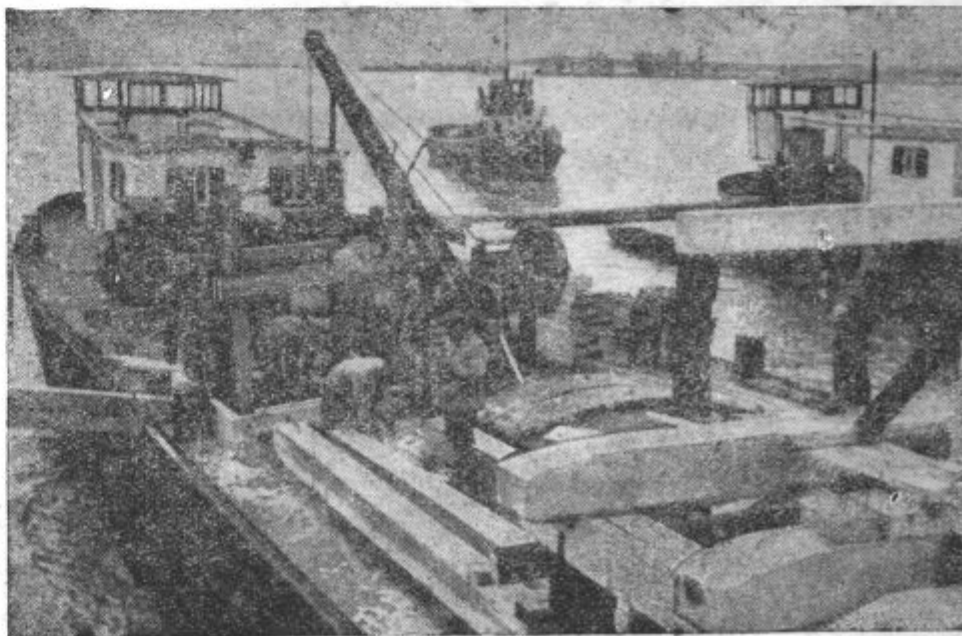
Nemške priprave za postavitve mostu čez Donavo
