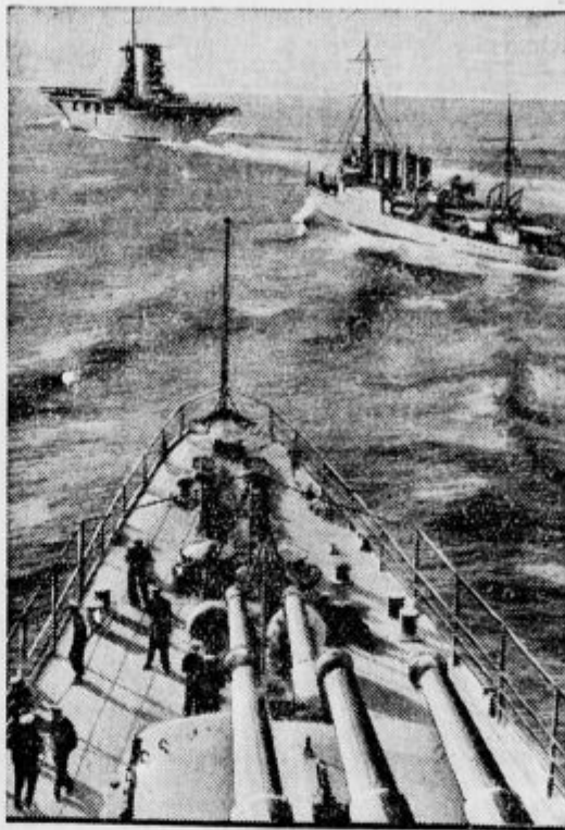
Prizor z letošnjih jesenskih vaj ameriške mornarice pri Los Angelesu. V ozadju vidiš ladjo matico »Saratoga« za letala, sledi ji križarka »Bromes«, spredaj topovi na bojni ladji »Pensacola«.
