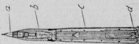
a) vžigalna glava, b) izstrelak, c) tulec, d) vžigalna kapa
