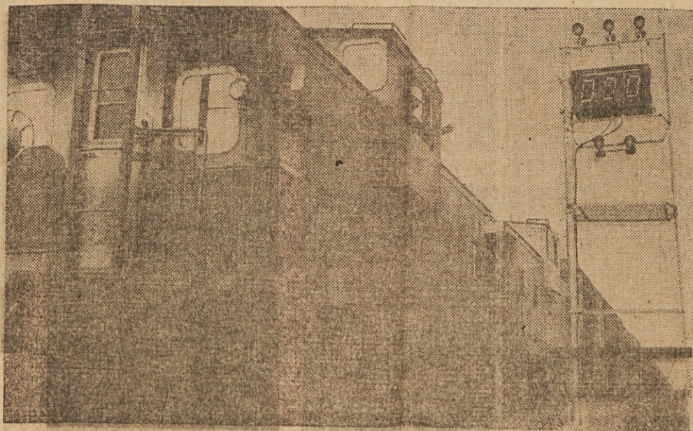
ELEKTRONSKI PREGLED — Na Burlington-Northern železnici so namestili elektronske naprave, ki nadzirajo ležaje koles na vozovih mimoitečih vlakov. Če bi bil imel kak voz vroč ležaj, bi naprava pokazala to s številkami. Ničle pomenijo, da je vse v redu.
