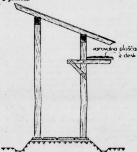
Sl. 5. Podrobna izvedba sušilne lope.
