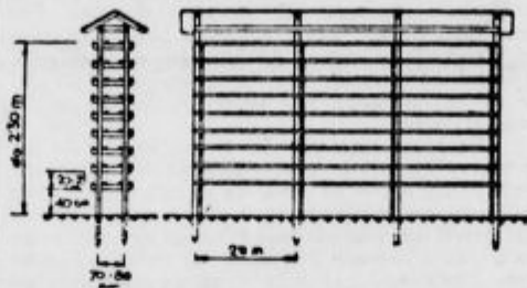
Sl. 6. Kozolec za sušenje.
