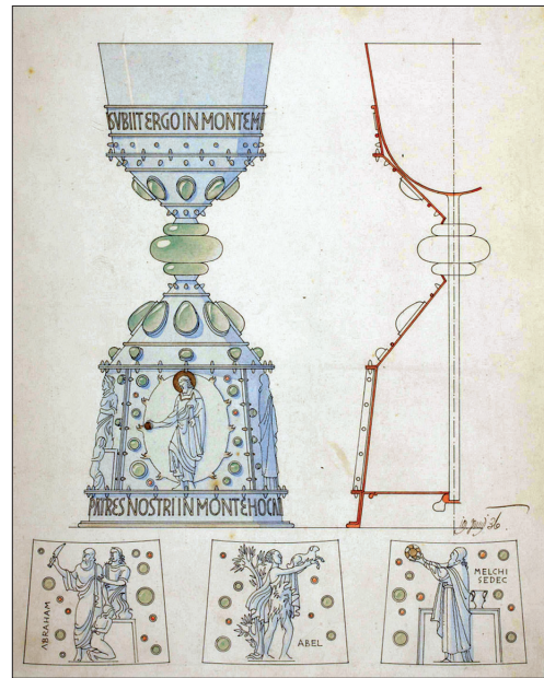
Plečnikov načrt za Omanov kelih, 19. junij 1936
