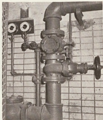
Sprinkler naprave so po 95 letih delovanja še vedno uporabne.
