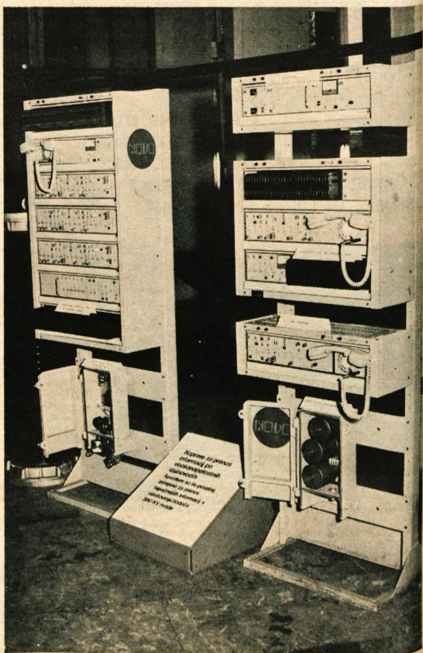
Naprave za prenos informacij po visokonapetostnih dalnovodih. Posebej so prirejene za prenos informacij v obratovanju bodoče 380-kilovoltne mreže
