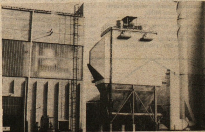
KURILI BODO LUBJE — V tem kotlu v TCP Videm kurijo ljubje. Vsako leto bodo prihranili 750.000 dolarjev ali 25.000 ton lignita, v zrak pa bo šlo 300 t manj žvepla. (Foto: J. Simič)
