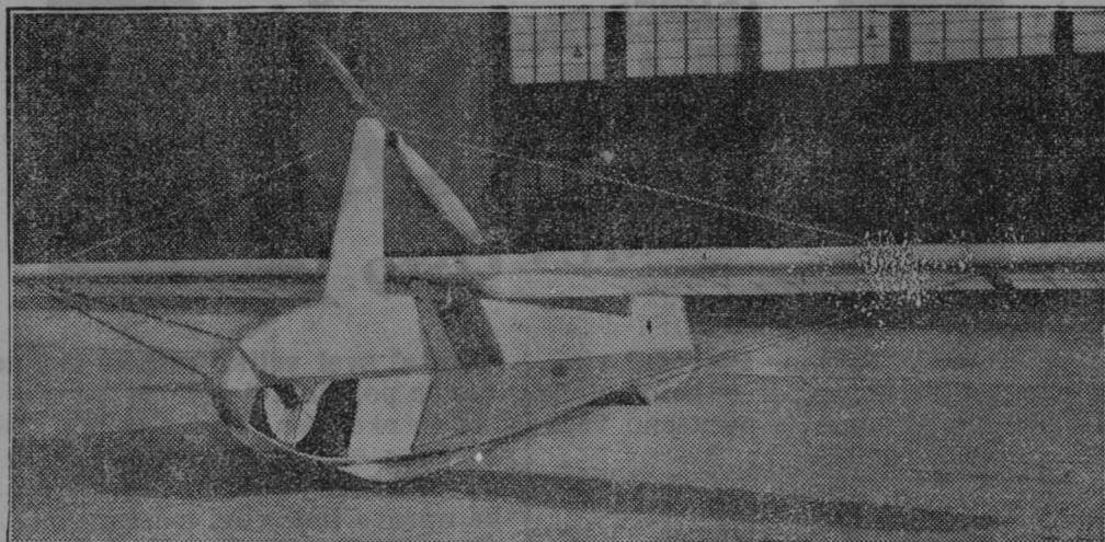
Prvo letalo na pogon z nogami brez motorja. Na tem letalu je preletel Nemec Dünnebell razdaljo 235 m 1 m visoko.
