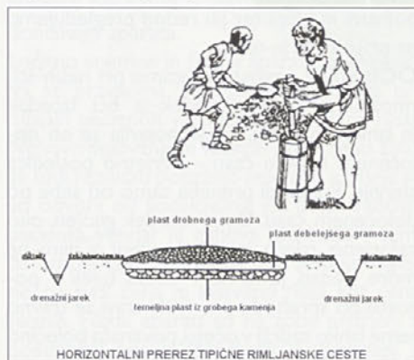
HORIZONTALNI PREREZ TIPIČNE RIMLJANSKE CESTE
