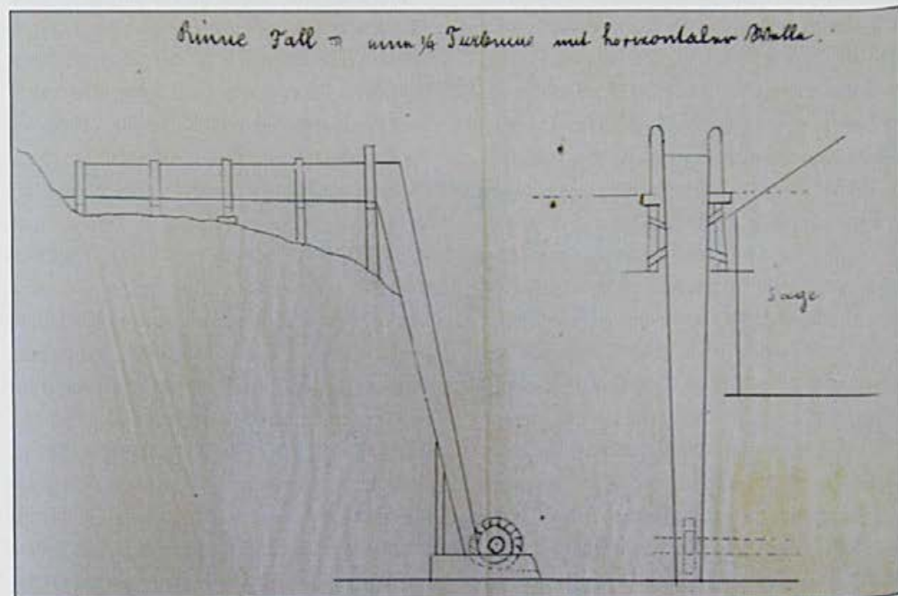
Za žago je predvidena enočetrtinska turbina z vodnim padcem 8 metrov. Foto: arhiv Vincenca Demšarja
