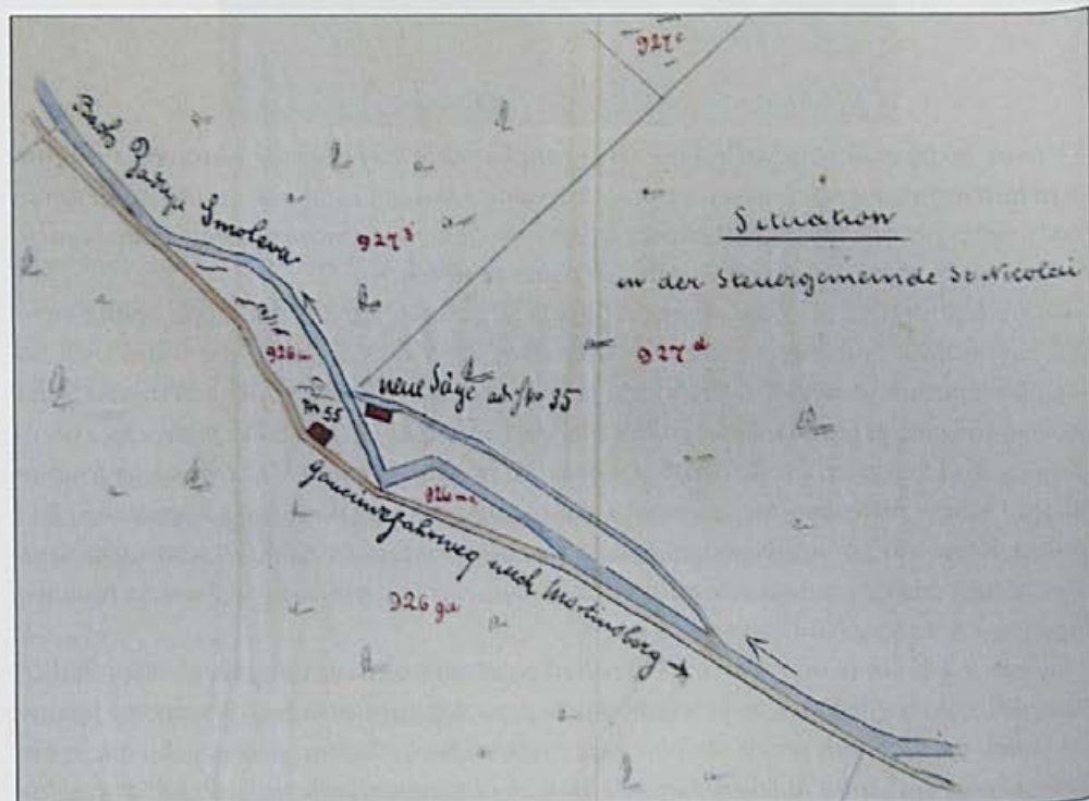
Situacijski načrt nove Javhove žage. Foto: arhiv Vincenca Demšarja
