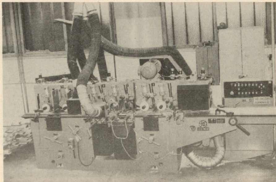
Še eden od glavnih strojev v Mizarstvu – štiristranski skobeljnik
