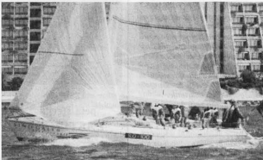
Šolska ladja Sinji galeb - prvo plovilo Obalne obrambe. Dolga je 13,2 m, jambor je visok 23 m, njena skupna teža znaša 7 ton.
