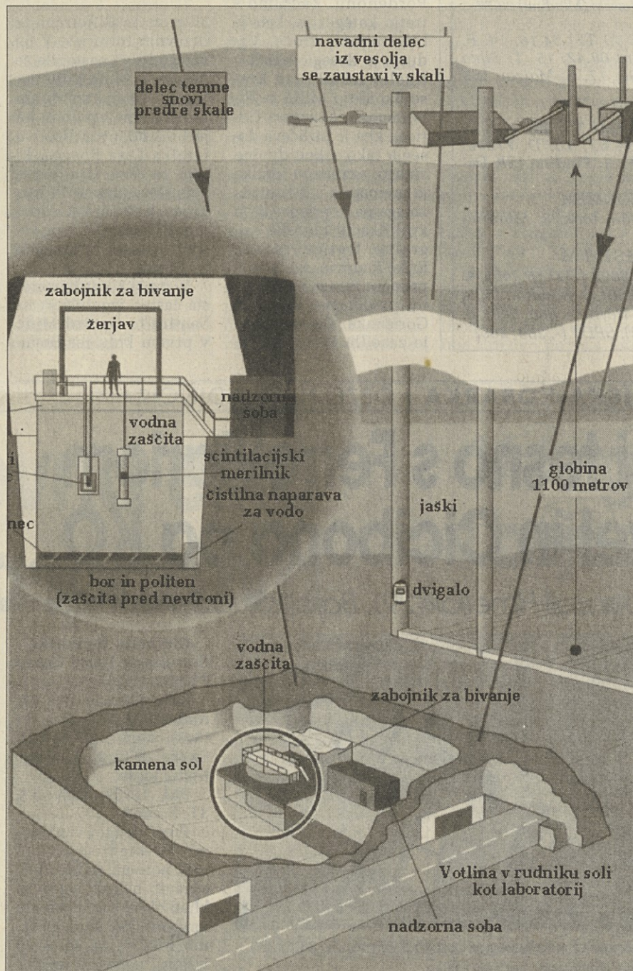
Naprave v angleškem laboratoriju za zaznavanje delcev temne snovi.
