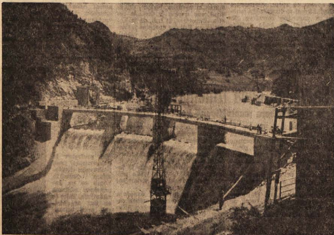
Jez hidrocentrale Jajce II.
