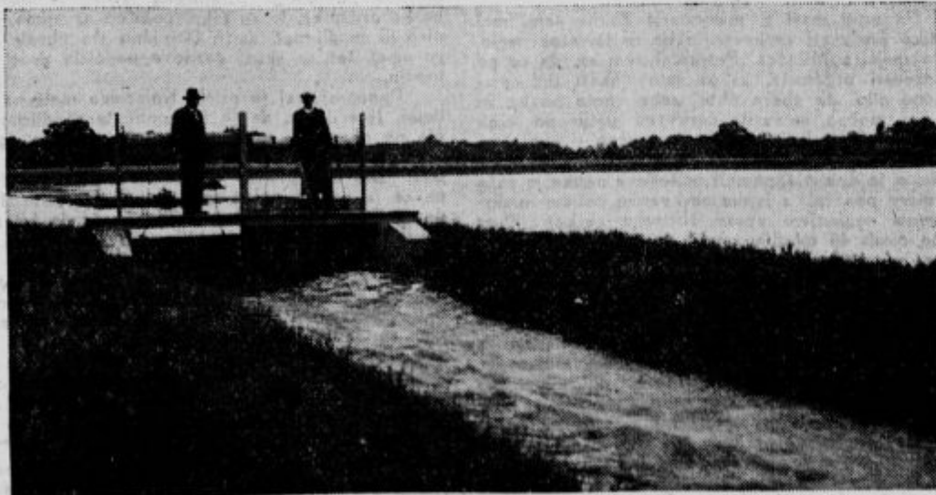
Namakalna naprava na obsežnih šolskih travnikih kmetij. šole v Rakičanu. V ozadju vidimo razsežen travnik, ki je ves zalit z vodo, v ospredju pa odprto zatvornico, skozi katero se odteka izčiščena voda po odtočnem kanalu v strugo Lendave.
