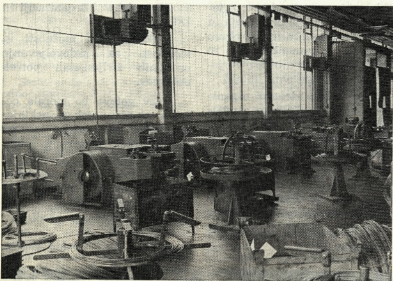
Skupina strojev za stiskanje vijakov in zakovic
