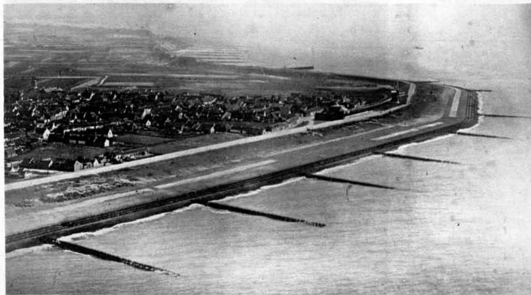
Pogled na obrežne nasipe na Nizozemskem.
