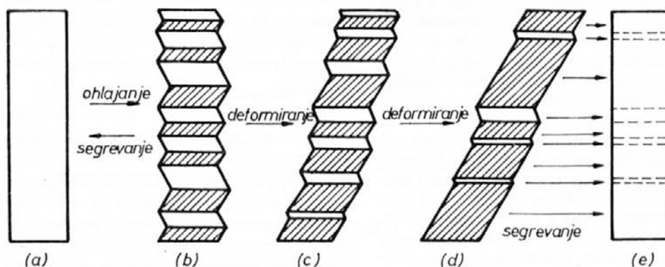
Sl.3: Shematski prikaz preorientacije in ponovne spremembe oblike; (a) in (c) sta beta fazi
