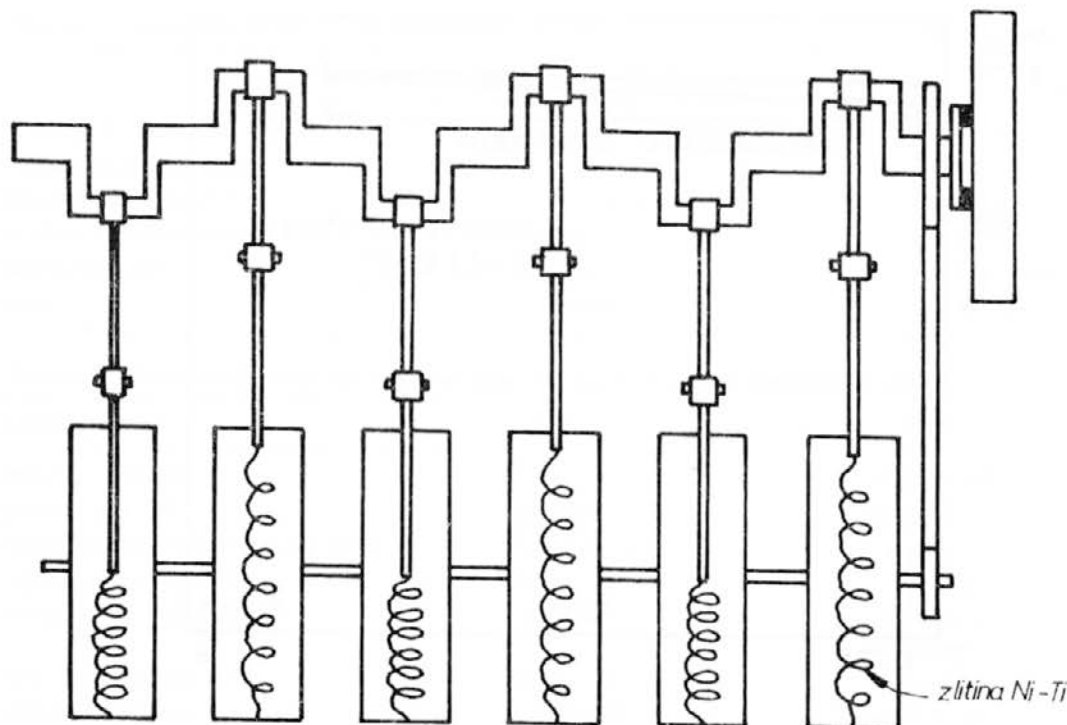
Sl.6: Toplotni stroj z elementi, ki si zapomnijo obliko
