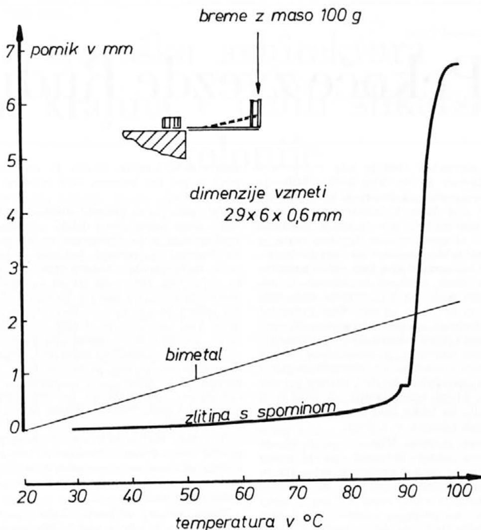
Sl.5: Karakteristika elementa, ki si zapomni obliko, in bimetala
