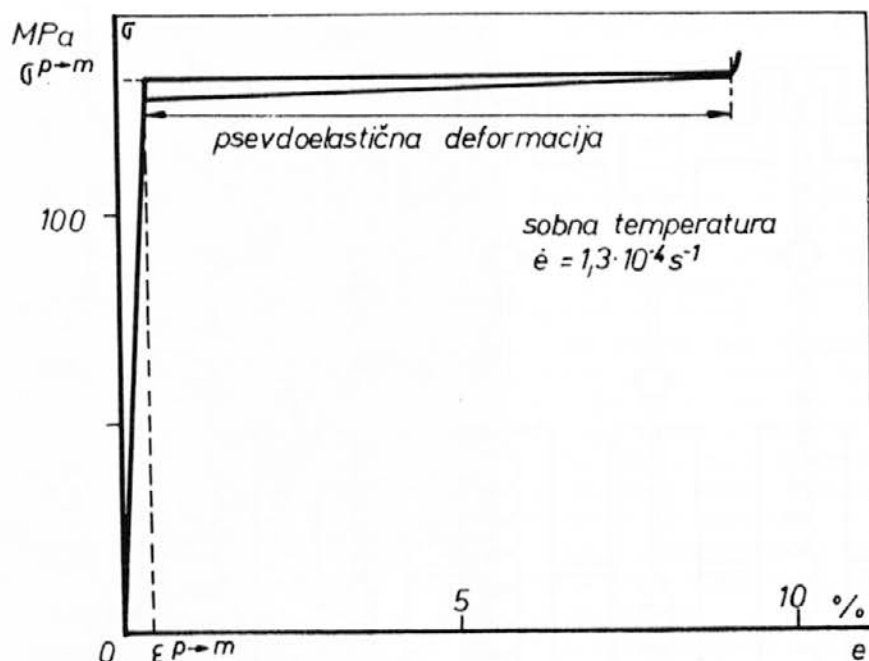
Sl.4: Psevdoelastična deformacija beta monokristala z dano orientacijo
