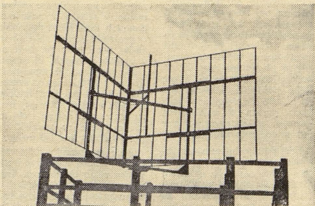
Antena dipol pred kontrolnim reflektorjem. To 147 kg težko anteno so izdelali v laboratoriju za antene ZZA po naročilu podjetja za distribucijo električne energije Elektro — Ljubljana
