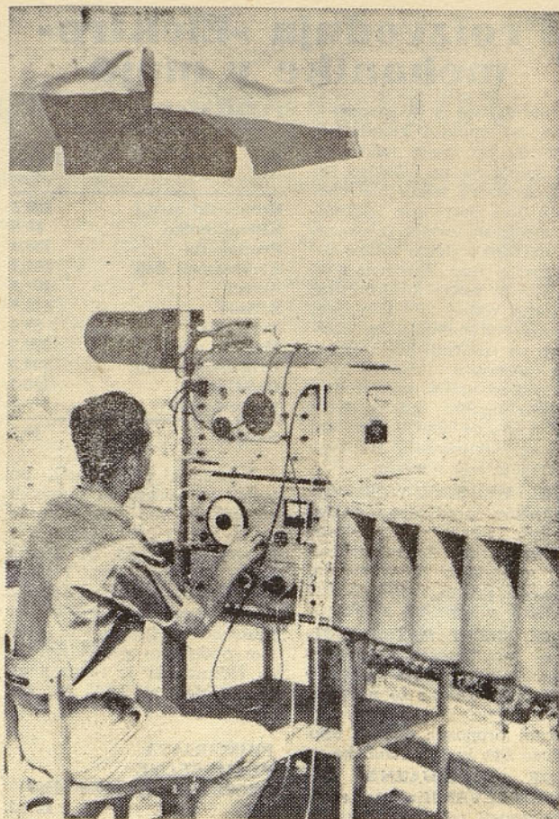
Laboratorij za antene ZZA dela največ za tovarno elektronskih naprav v Stegnah pri Ljubljani. Slika prikazuje končno kontrolno merjenje anten na ravni strehi petnadstropne stavbe, kjer ima laboratorij svoje merilno mesto. Načrte za te antene so izdelali v laboratoriju za antene ZZA, sedaj pa jih serijsko izdeluje TEN
